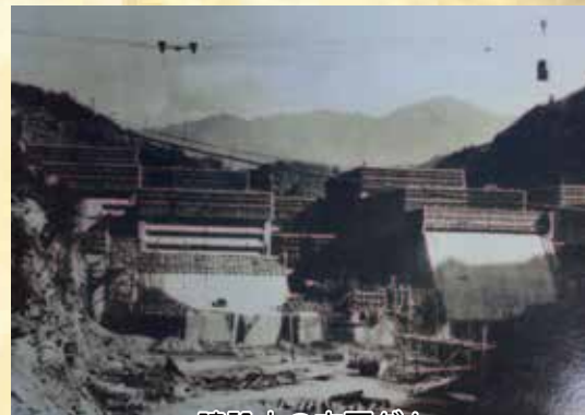
建設中の市房ダム
